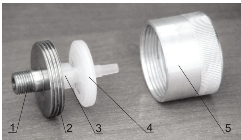
Рис 5. Пробоотборное устройство.
