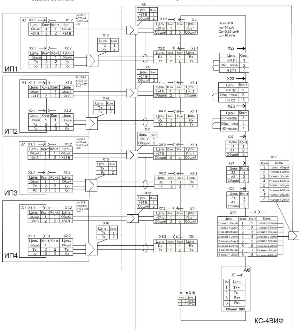
Рис. 10. Схема подключения ИП к блоку KS Клеммник X18 – подключение питания 220 В, 50 Гц Клеммники X20, X21 – подключение KS по интерфейсу RS-485 к ПК или блоку БГЕ, разъем X1(A6) – подключение KS к ПК или к блоку БК по линии Ethernet / Internet, клеммник X27 – подключение KS к блоку БР; разъем X29(внутренний) X17 (внешний) – токовый выход (см. Приложение 6)
