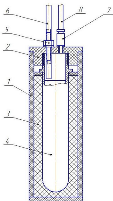
Рис. 1. Устройство для очистки фотоионизационного детектора
